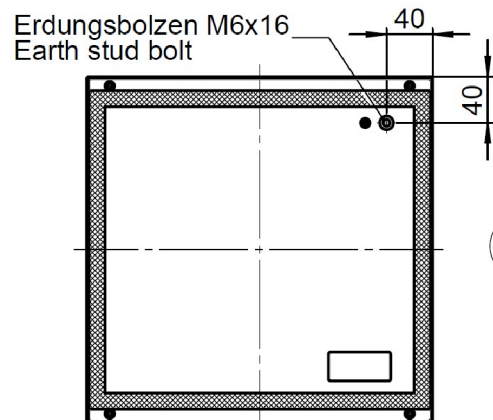
Deckel / Lid
