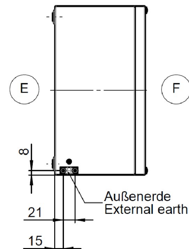
Senkschraube Lens head screw M5 DIN 966
