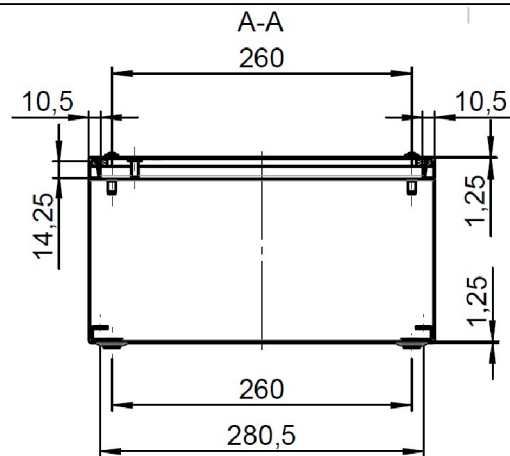
Unterteil / Base
